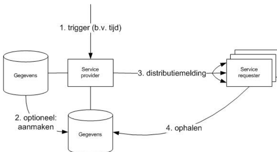
Figuur 5 Use case '(multi-) distributie'
