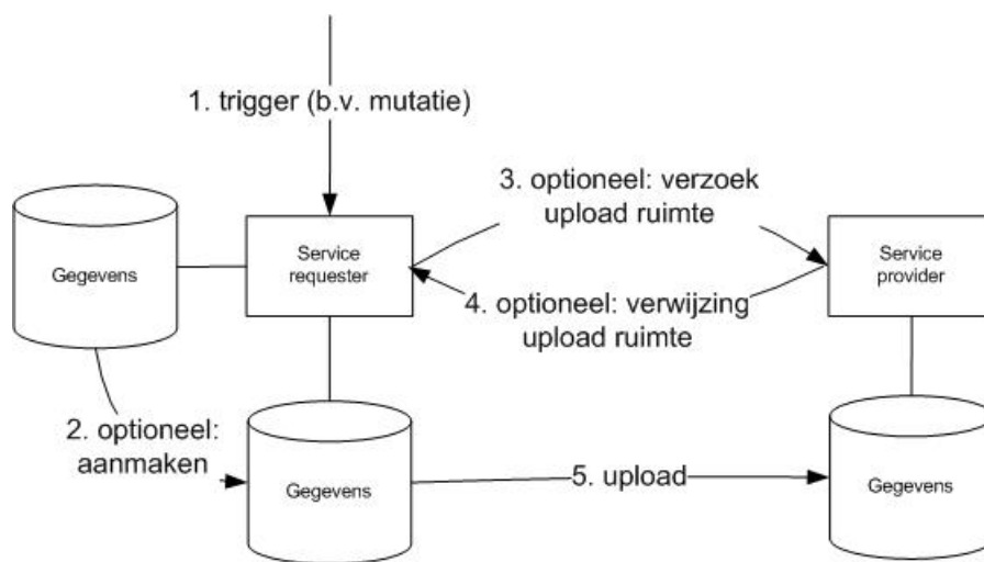
Figuur 6 Use case 'Upload'
