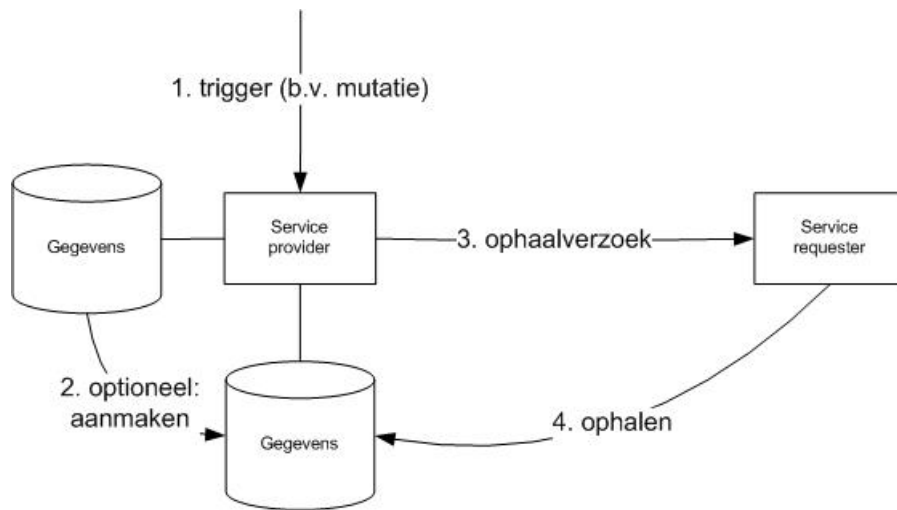
Figuur 4 Use case 'Verzending'
